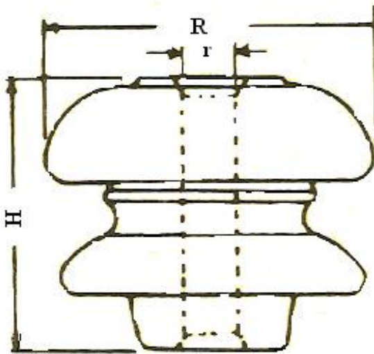
L. T. Shackle Insulator
