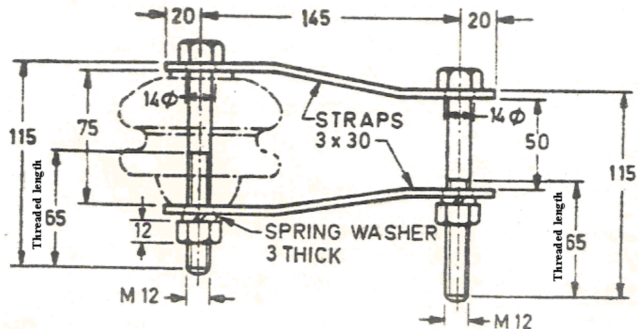
Fig-1 L.T.STRAP& BOLTS
