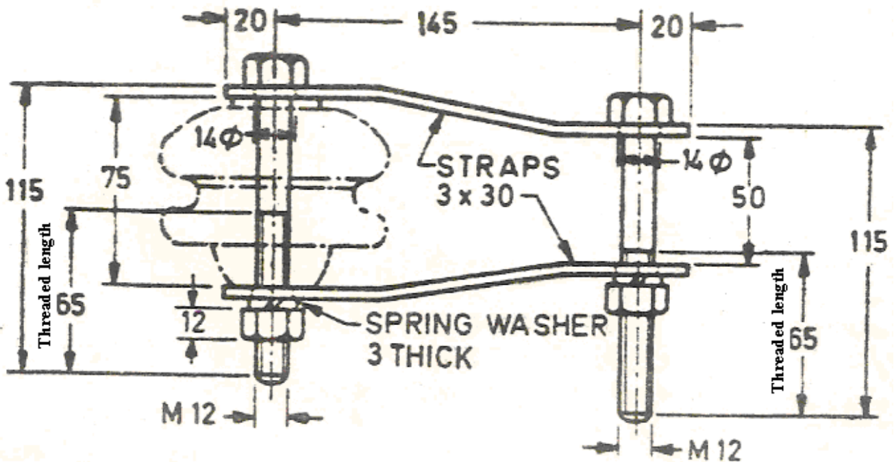
Fig-1 L.T.STRAPS & BOLTS
